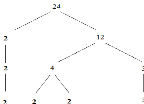
Figura 1: Árvore de decomposição do 24.
